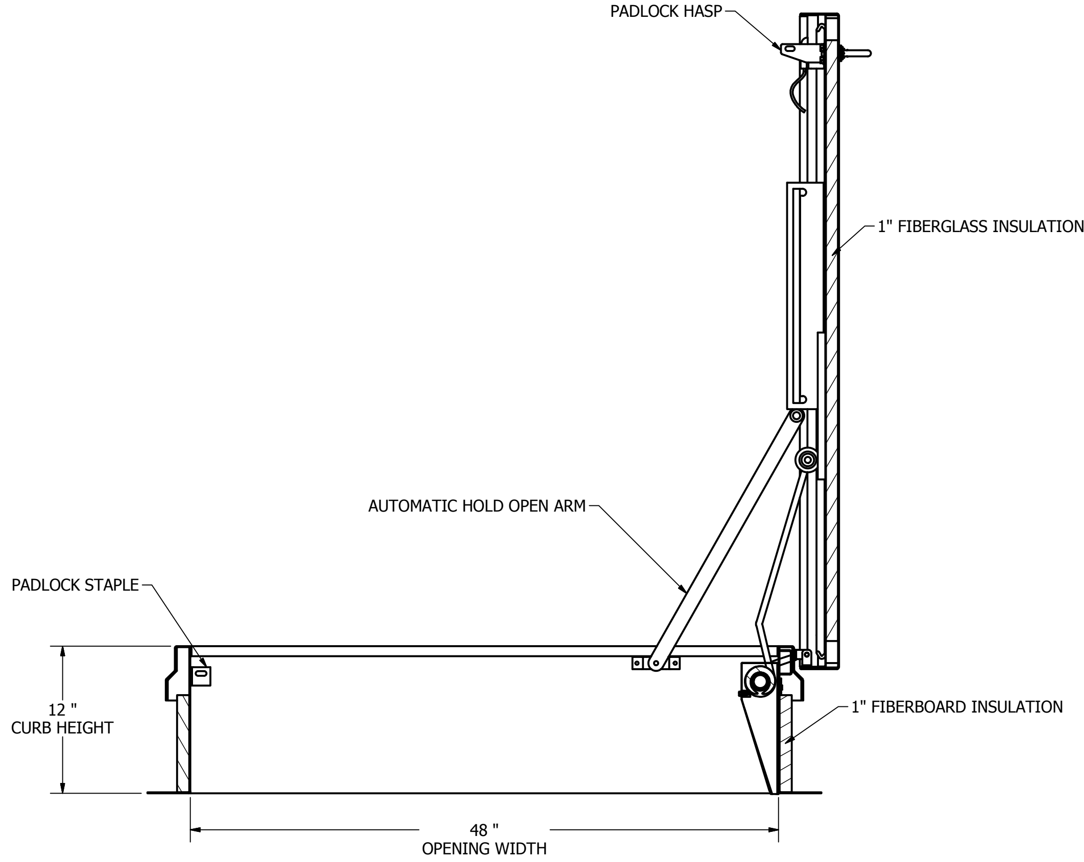
SECTION A-A
